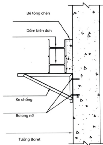
Dầm biên đôi (Loại 2)
