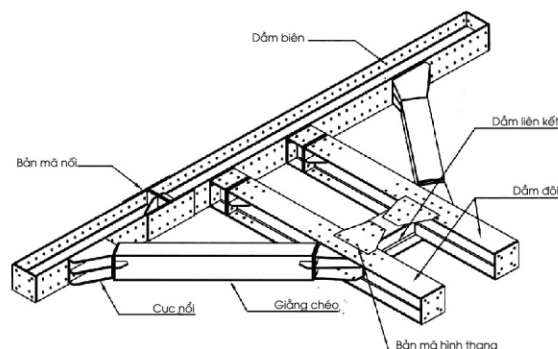
Hình minh họa B: Liên kết giằng chéo với dầm đôi
