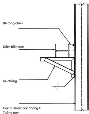
Dầm biên đơn
