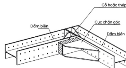
Cục chặn góc khi dầm biên cùng cao độ
