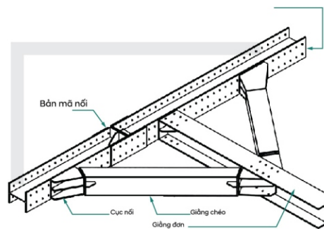
Hình minh họa A; Liên kết giằng chéo với dầm đơn
