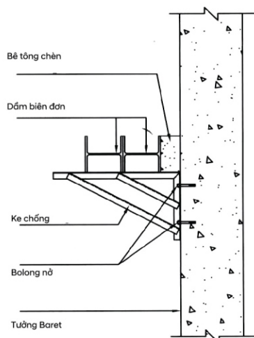
Dầm biên đôi (Loại 1)
