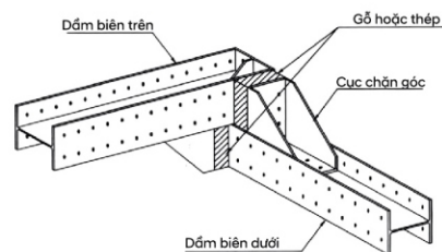
Cục chặn góc khi dầm biên khác cao độ
